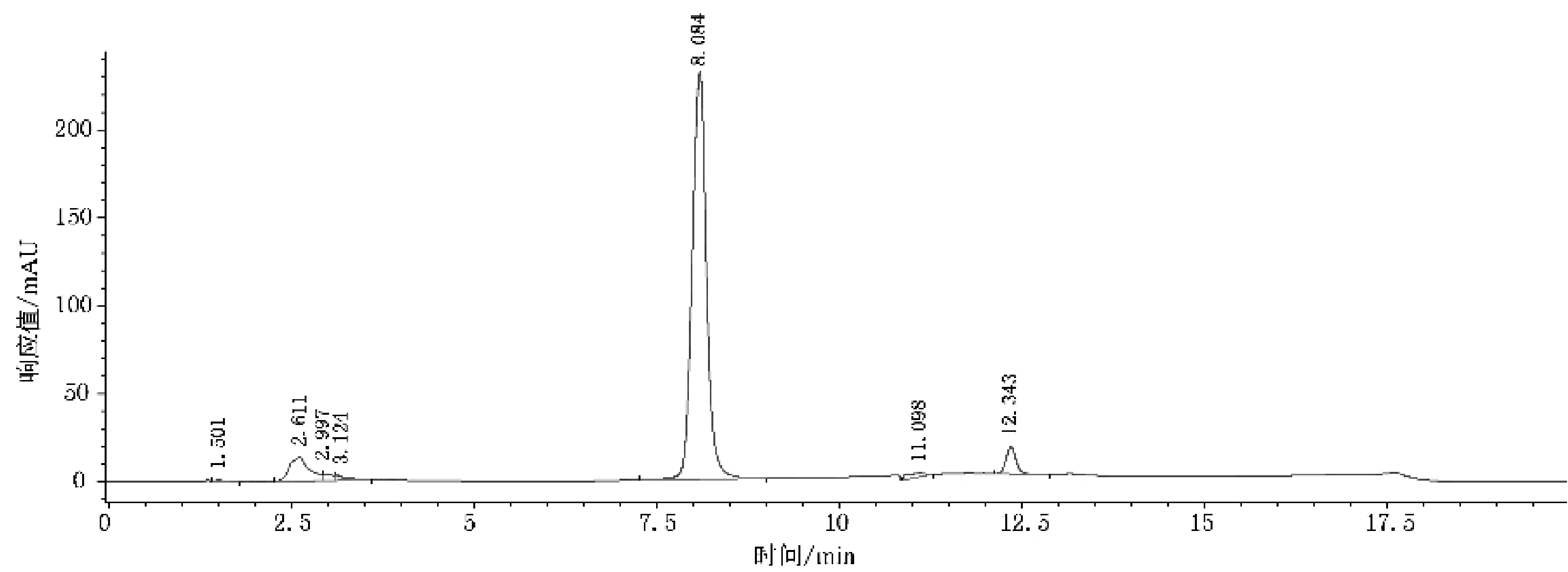
图 A.1 L-抗坏血酸-2-单磷酸酯盐标准溶液(100 µg/mL)色谱图
